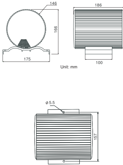
尺寸 (单位: 毫米)
