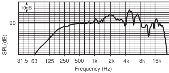
频率响应
