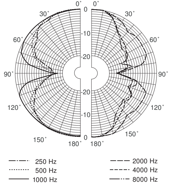
指向性图
